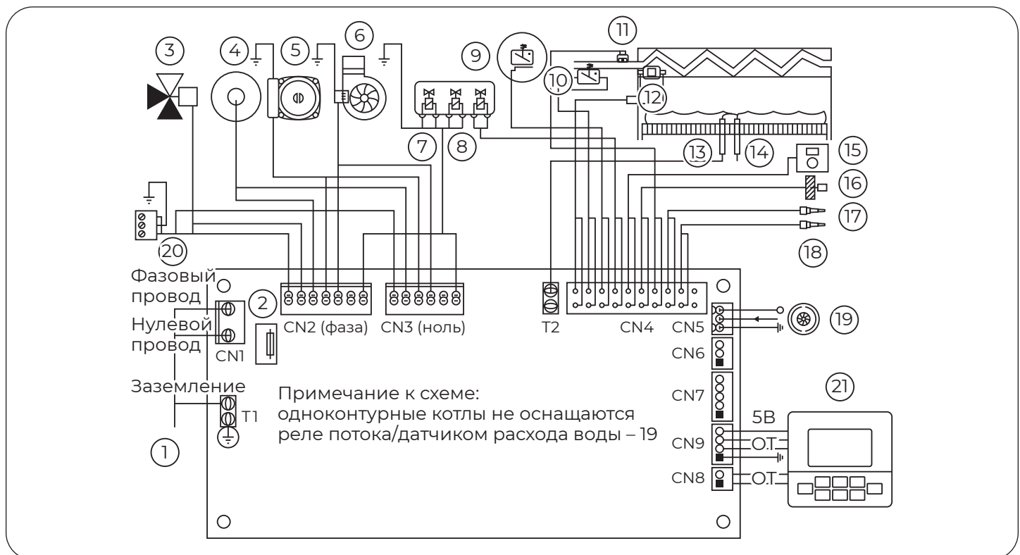
Рис. 31. Электрическая схема.
