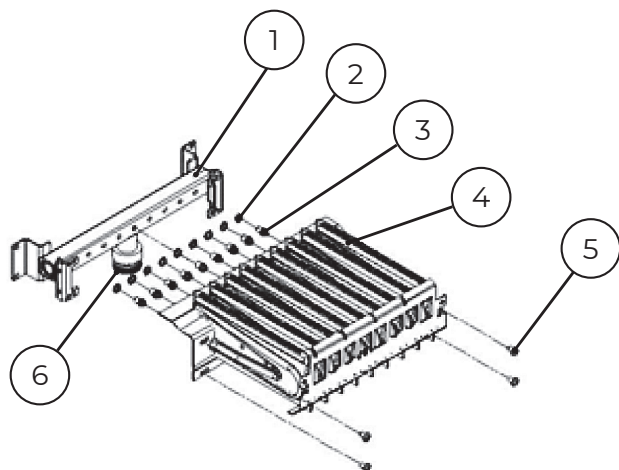
Рис. 24 Газовая горелка.
