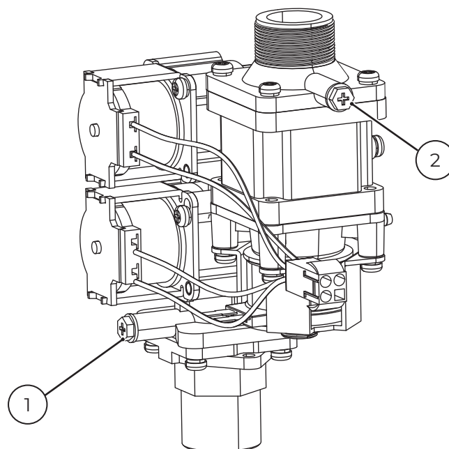
Рис. 25. Газовый клапан.
